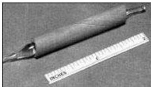
Capsule contenant de l'acide sulfurique encastré dans un tube en caoutchouc pour protection
