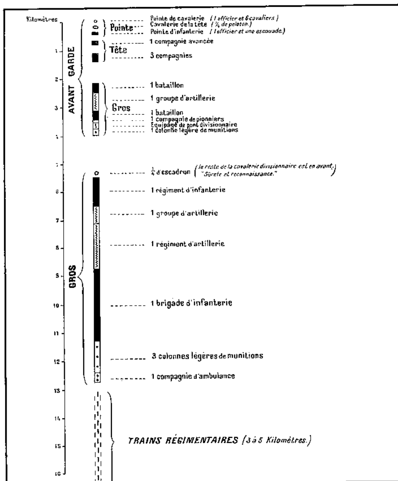
SCHEMA INDIQUANT L'ORDRE DE MARCHE D'UNE DIVISION ALLEMANDE
