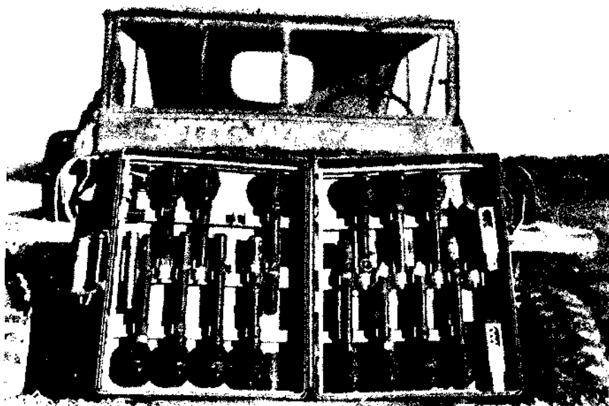
Figure 20.—Special projectile 361 for signal pistol ( Wurfkörper 361 für Leuchtpistole ).
