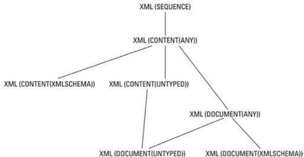
FIGURE 2.1 Les relations entre les sous-types XML.
