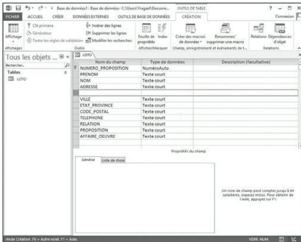
FIGURE 4.8 La fenêtre de création de la table après avoir rajouté un emplacement pour une seconde ligne d'adresse.
