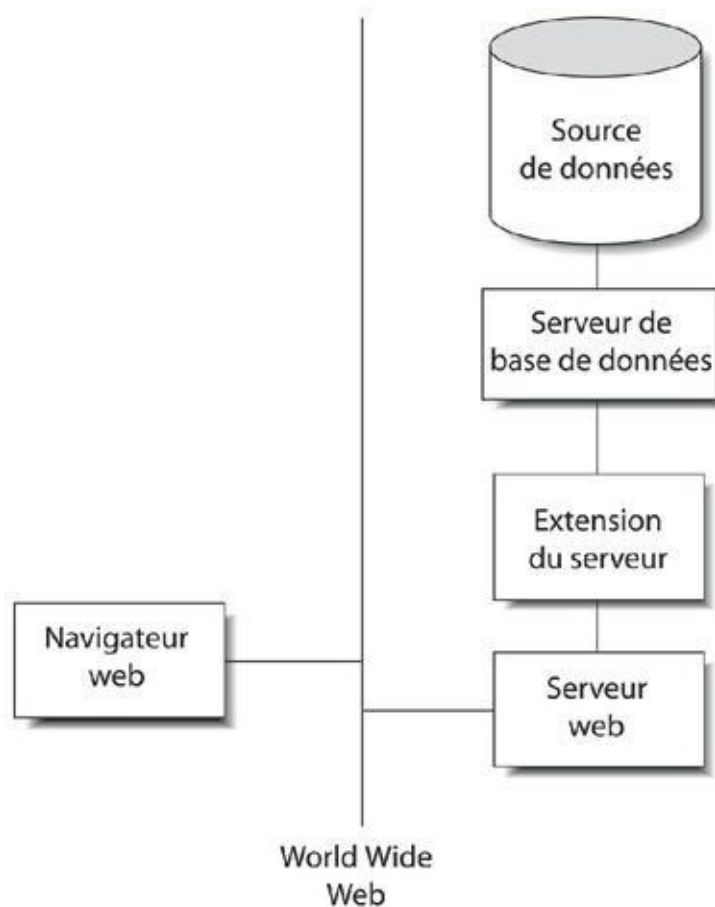
FIGURE 17.2 Système d'accès à une base de données sur le Web dotée d'une extension serveur.
