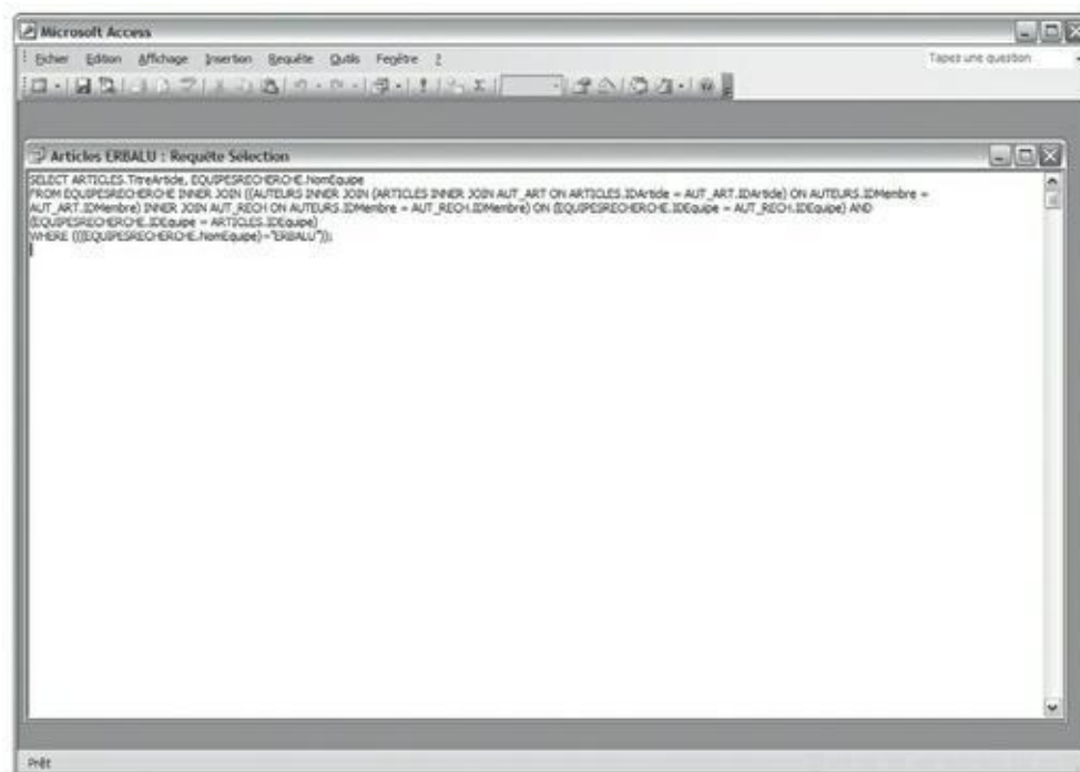
FIGURE 16.3 Une instruction SQL qui sert à retrouver les noms de tous les articles écrits par des membres de l'équipe ERBALU.
