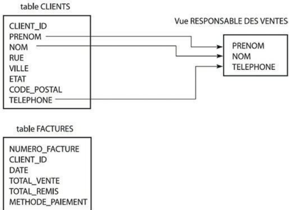
FIGURE 1.4 La vue du RESPONSABLE DES VENTES dérive de la table CLIENTS.
