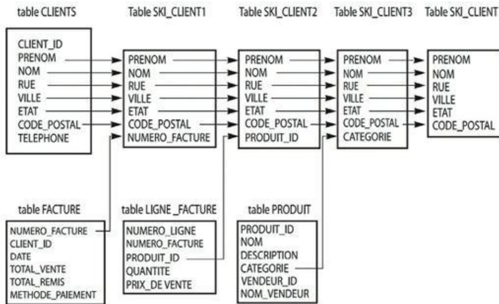
FIGURE 3.4 La création d'une vue multitable en utilisant des jointures.
