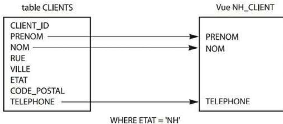
FIGURE 3.2 Vous dérivez la vue NH_CLIENT de la table CLIENTS.
