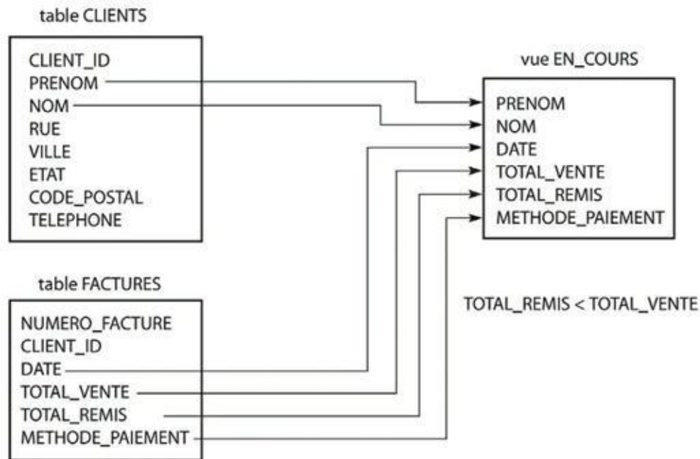
FIGURE 1.6 La vue EN_COURS tire ses données de deux tables.
