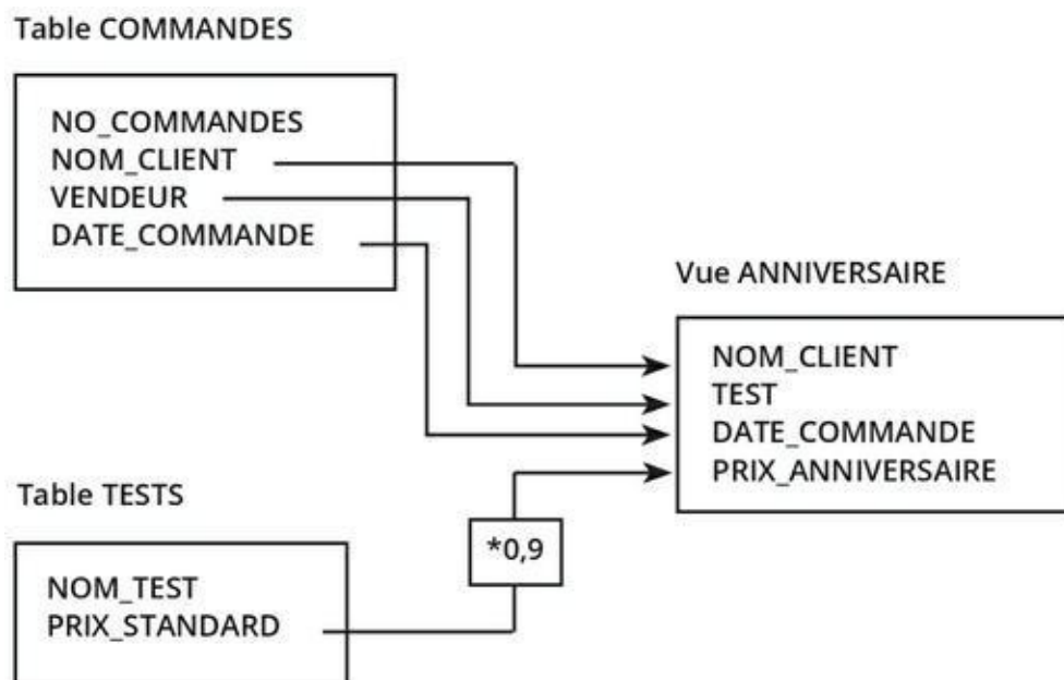
FIGURE 6.3 La vue créée pour afficher les prix anniversaire.
