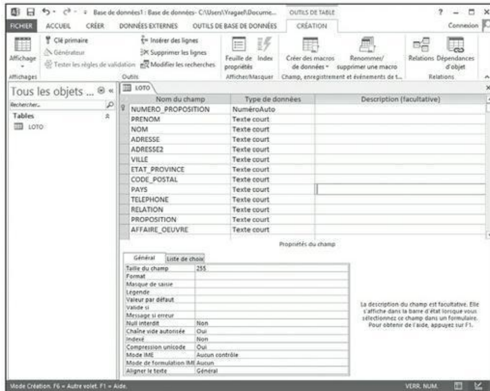
FIGURE 4.9 Votre table révisée devrait ressembler à ceci.
