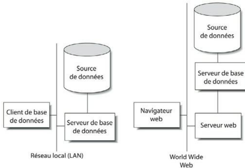
FIGURE 17.1 Système client/serveur versus système de base de données sur le Web.
