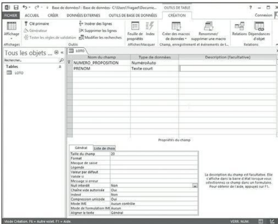
FIGURE 4.5 La fenêtre de création de la table une fois que vous avez défini Prénom.
