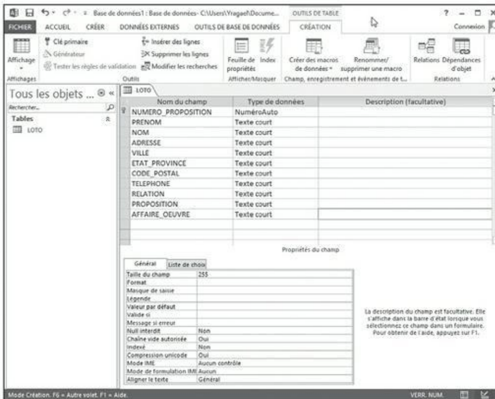
FIGURE 4.7 La fenêtre de création de la table une fois que tous les champs ont été définis.
