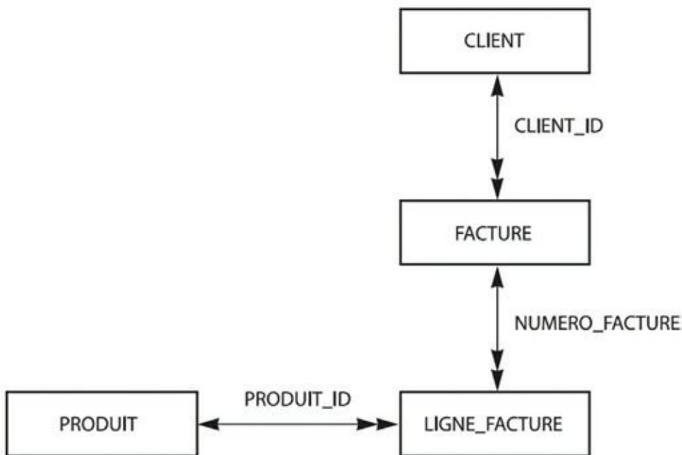
FIGURE 3.3 La structure de la base de données du magasin de sport.
