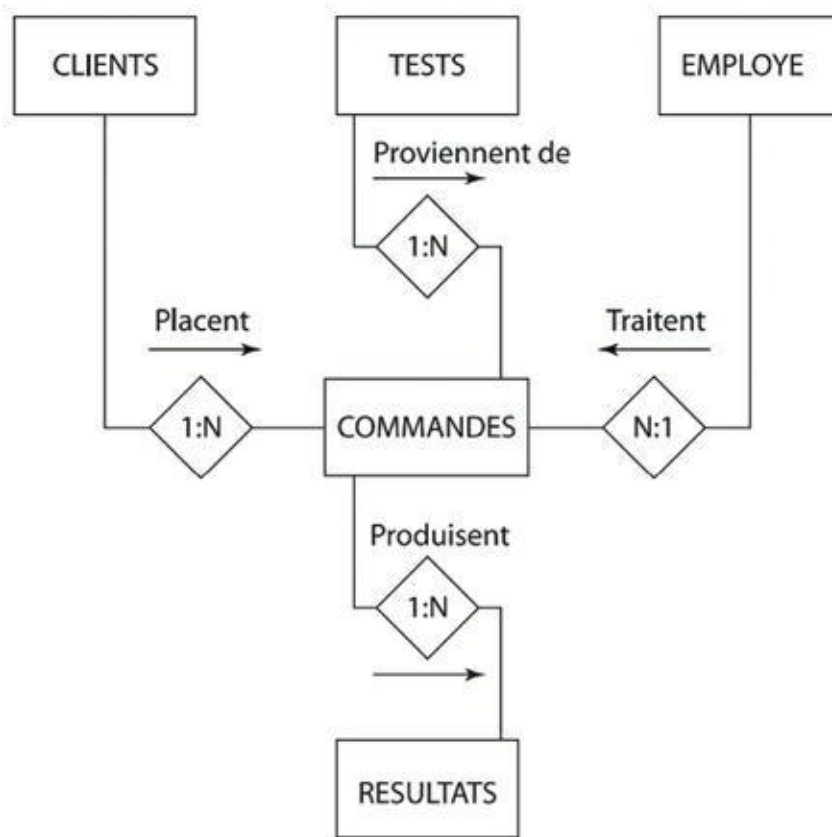
FIGURE 5.1 Les tables de la base de données de VetLab.
