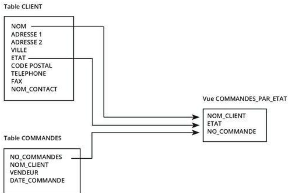
FIGURE 6.1 La vue COM-MANDES_ PAR_ETAT pour le responsable marketing.
