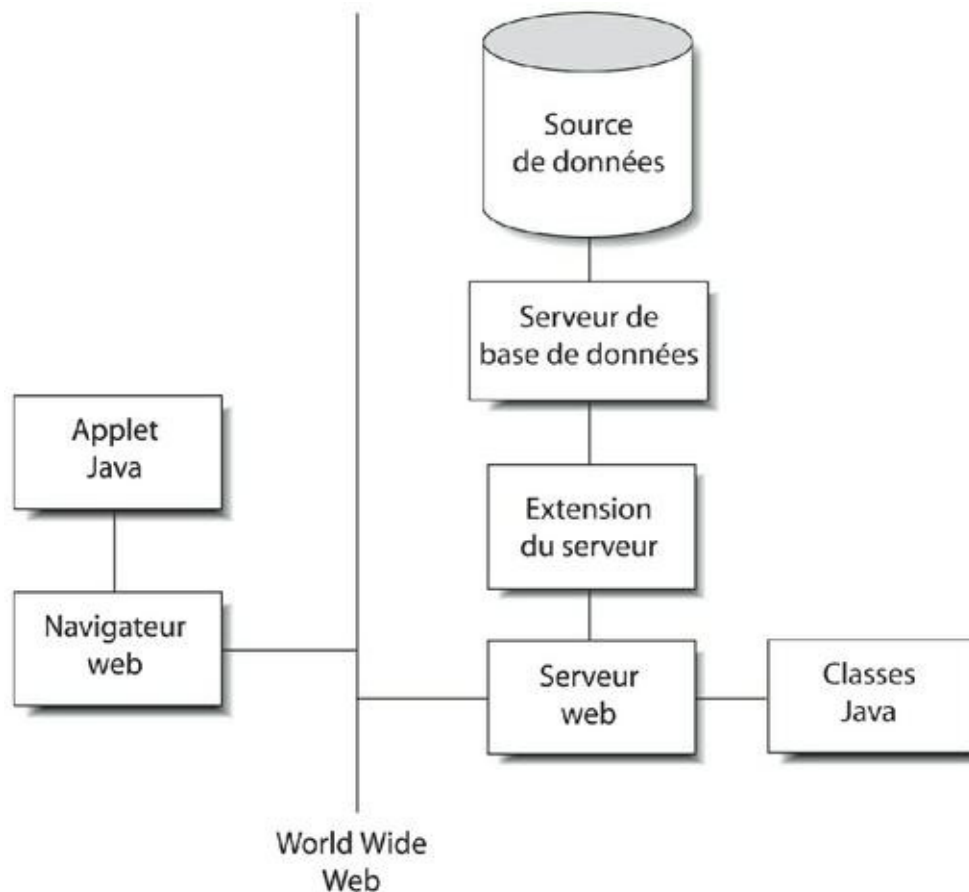
FIGURE 17.3 Application de base de données pour le Web utilisant une applette Java.
