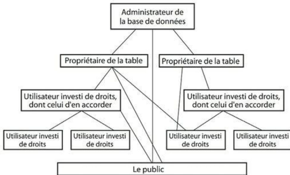
FIGURE 14.1 Hiérarchie des utilisateurs en fonction des privilèges d'accès.
