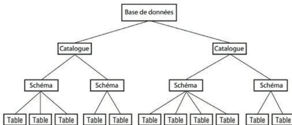
FIGURE 3.5 La structure hiérarchique d'une base de données SQL.
