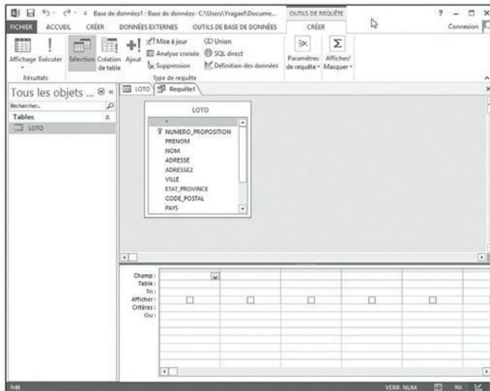
FIGURE 4.11 L'écran Requête une fois la table LOTO sélectionnée.
