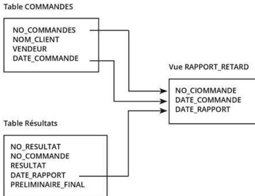
FIGURE 6.2 La vue RAPPORT_RE-TARD pour le responsable qualité.
