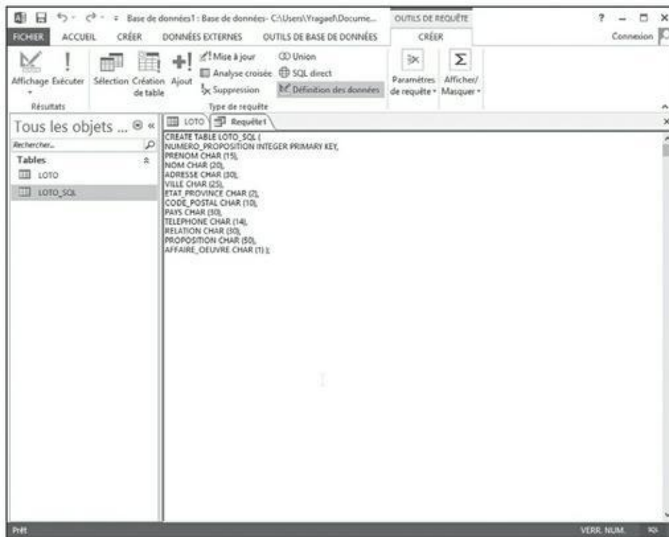
FIGURE 4.15 Création de la table LOTO_SQL.
