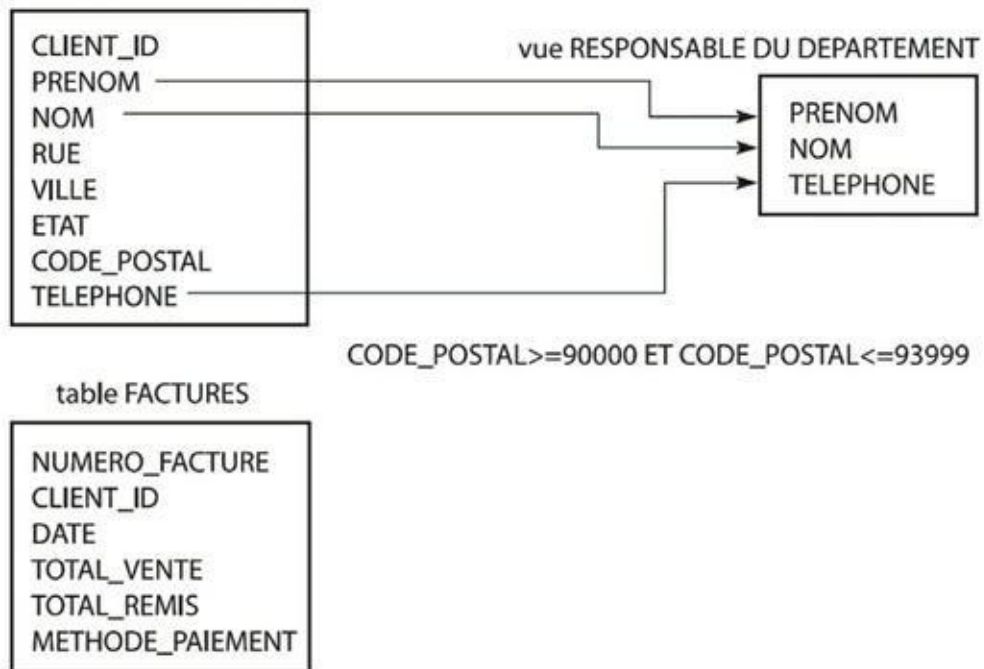
FIGURE 1.5 La vue du RESPONSABLE DU DEPARTEMENT ne contient que quelques-unes des lignes de la table CLIENTS.
